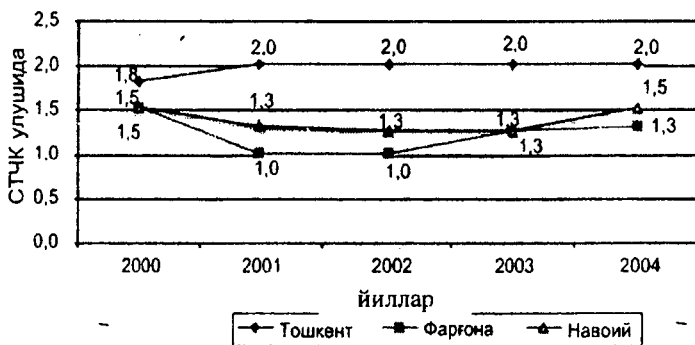
10-расм. Атмосфера ҳавосининг азот диоксида билан ифлосланганлик даражаси динамикаси
