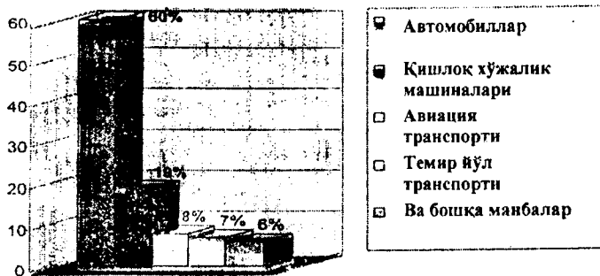
9-расм. Ўзбекистон республикаси бўйича ифлослантувчи моддалар ташланиши динамикаси, 2004-2006 йиллар (харакатланувчи манбалар).
