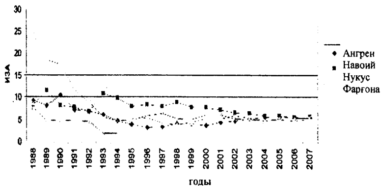
6-расм. Атмосфера ҳавосининг чанг билан ифлосланганлик даражаси динамикаси.
