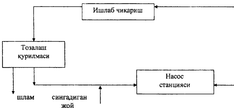
3-расм. Сув айланишининг кўриниши.
