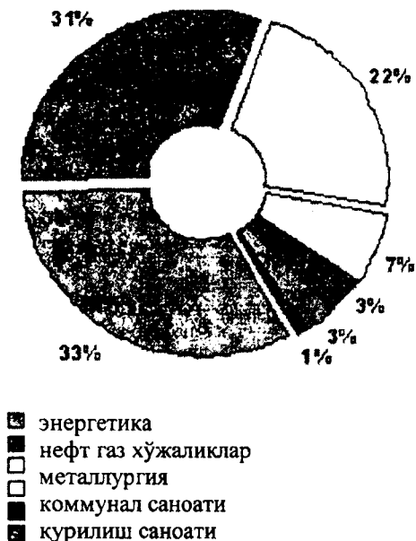
5-расм. Ўзбекистон Республикаси бўйича атмосфера ҳавосига ифлослантирувчи манбаларнинг улуши.
