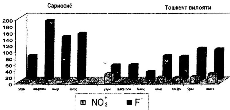
12-расм. Тошкент ва Сурхондарё вилоятлари ҳудудда ўсимликлар барглари таркибид мавжуд бўлган нитрат ва фторидлар (г/кг) (2001 -2003 ) йиллар.
