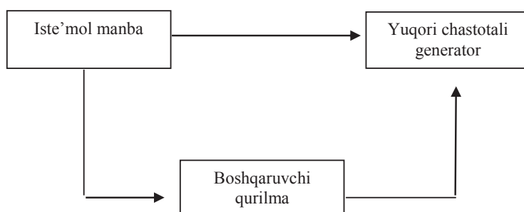
1-Rasm. Radiouzatuvchi qurilma blok-sxemasining tuzilishi
