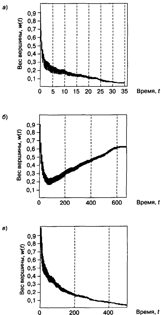
Рис. 2.2.3. Графики изменения основного показателя системы с управляющим воздействием
