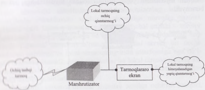
8.13-rasm. Himoyalangan yopiq va himoyalanganmaydigan ochiq qism-tarmoqli sxema.
