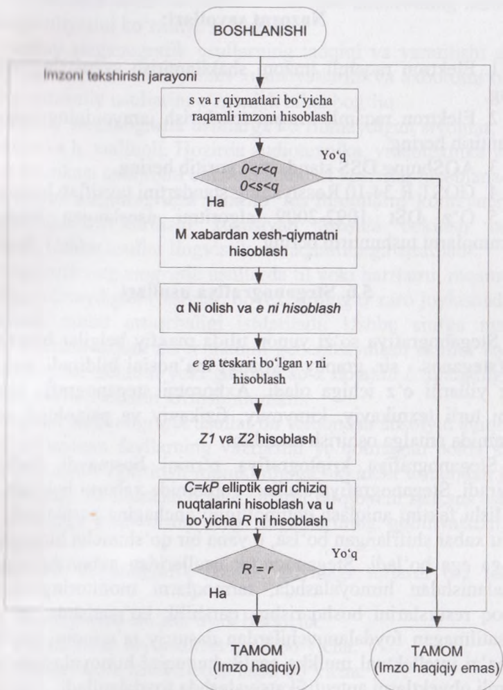
3.24-rasm. Elektron raqamli imzoni tekshirish jarayoni.
