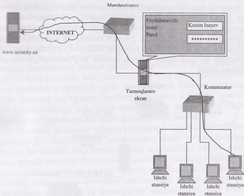
8.3-rasm. Parol bo'yicha foydalanuvchini autentifikatsiyalash sxemasi.
