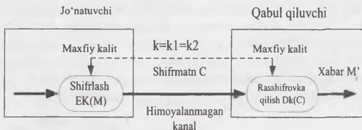
5.9-rasm. Simmetrik shifrlash kriptotizimining sxemasi.
