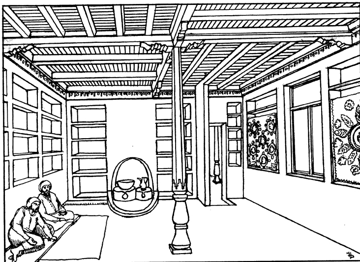
37-расм. Тошкент вилояти. Четсув тоғ қишлоғи. Ҳанов уйида асосий хона ички кўриниши (муаллиф чизмаси).
