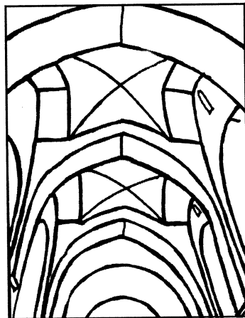
185-расм. Туркменистон, Анав масжиди. Калқонсимон равоқларга ўрнатилган гумбазлар тури (Г.А. Пуғаченкова бўйича).
