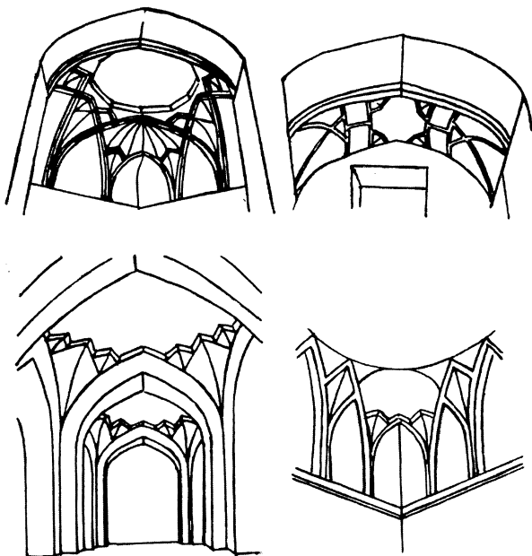
185-расм. Туркменистон, Анав масжиди. Калқонсимон равоқларга ўрнатилган гумбазлар тури (Г.А. Пуғаченкова бўйича).
