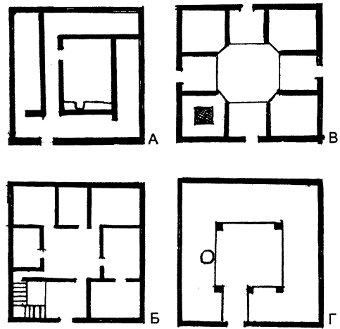
143-расм (схема). Турар жой иморати хоналарининг камайиб бориши ҳисобиға қатталашуви босқичлари. А. Бухоро воҳаси. Турар жой тарҳи (милоддан аввалги III-аср). Б. Қиз қалъа. Иккинчи қават тарҳи (VI- VIII асрлар). В. Марв. Турар жой иморатининг иккинчи қавати (XI- XII асрлар). Унда тўрт томон марказий ўқларидаги айвонлар ҳисобиға очқликка эришишға ҳаракат қилинган. Г. Тоғли Бадахшон. XIX-XX асрларда қурилган турар жой иморатлариға хос андозавий тарҳ (муаллиф чизмаси).
