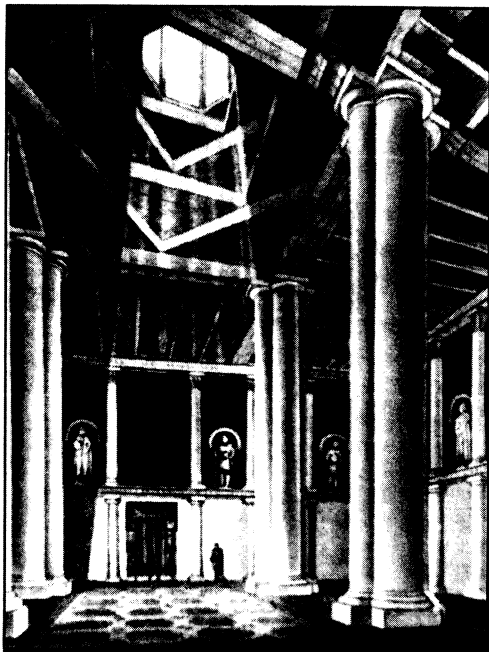
48-расм. Нисо. Сароининг томонлари тенг (квадрат) хонаси кури- ниши (Г.А. Пузаченкова реконструкцияси).
