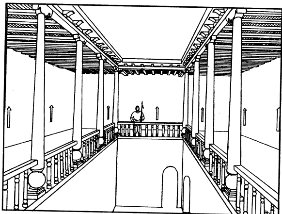
9-расм. Туркменистон. Бургут қалъа воҳасида VIII асрга оид кўшкнинг иккинчи қавати ички кўриниши Е.Е. Неразикнинг китобига мазкур қалъа иккинчи қавати "П" ҳарфи шаклида девор билан ўралган. Биз ўз реконструкциямизда қалъанинг шу қисмини айвон шаклида бердик. Е.Е. Неразикнинг ўзи ҳам қалъанинг иккинчи қавати булган, деб тахмин қилади (Неразик Е.Е., 1966, 70-б.).
