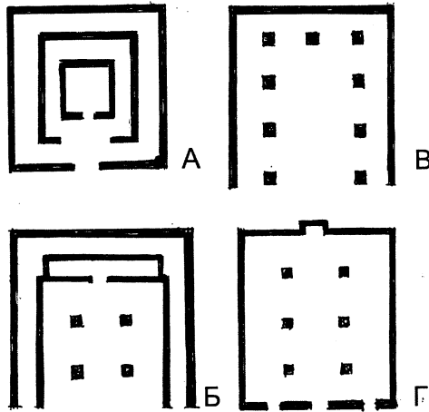
144-расм (схема). Марказий Осиё меъморчилиғида обида тарҳининг асрлар давомида ўзгариб бориши. А. Оқ- Бешим.Будда ибодатхонаси тарҳи (илк ўрта асрлар). Б. Панжикент. Ибодатхона тарҳи. Илк ўрта асрларда атрофи далон билан айлантирилган тарҳ турли иморатларда қўлланилган. Унда Оқ- Бешим ибодатхонаси каби иморатнинг марказий хонаси деворлари олиб ташланиб ўрниға устунлар ўрнатилган. В. Термиз шоҳлар саройи (ўрта асрлар). Унда асосий хона билан далон устунлар ёрдамида яхлит композицияға бирлаштирилган. Г. Сунғи ўрта асрларда шундай тарҳ диний ва маданий иморатларда кенг қўлланилган (муаллиф чизмаси).
