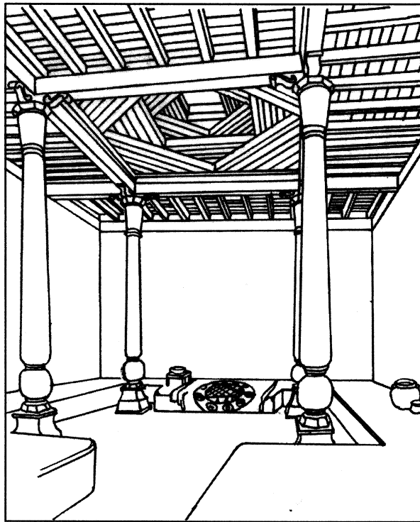
2-расм. Панжикент. Илк урта асрларда меҳмонхона ички кўриниши (В.Л. Воронина реконструкцияси).
