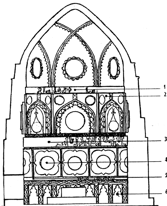
235-расм. Қирғизистон. Шоҳ-Фозил мақбараси қирқими. Мақбара ички қисми бўлинмалари тақсимоти (Д.Д. Иманқулов чизмаси). 1-қуфий ёзув билан тўлдирилган саккизбурчак юза; 2-равоқлар қавати; 3-ёзувли катта фриз; 4-кенг нақшли бўлинма; 5- қуфий ёзувли тор чизик; 6-изора.
