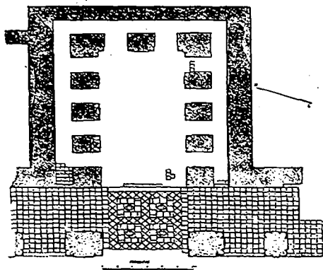
4-расм Термиз ҳолчимлари саройи қабулхонасининг тархи
