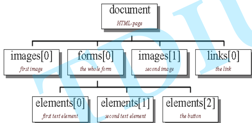
6.1-rasm. HTML-sahifa ob'ektlarining ierarxiyasi 50 .
