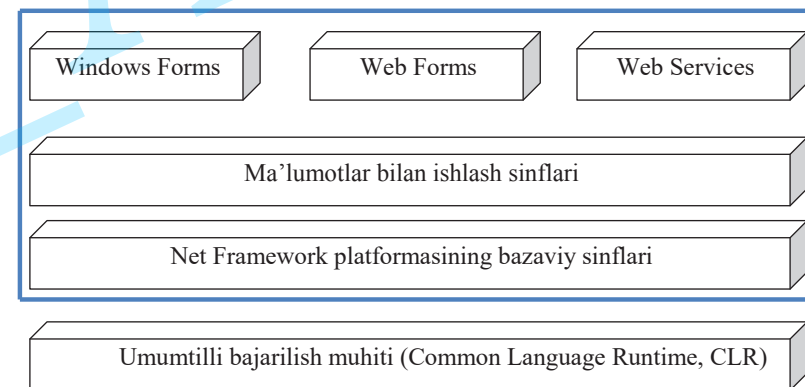
8.3-rasm. MS.NET Frameworkning arxitekturasi 69 .
