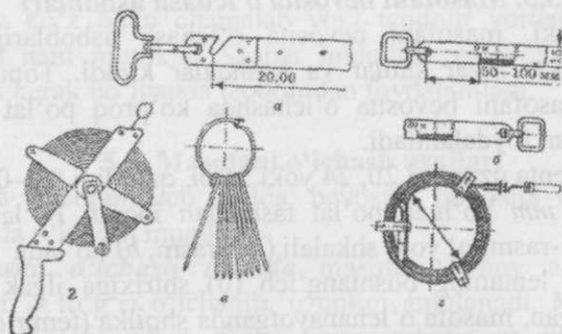
5.1-rasm. Masofa o'lchash qurollari Po'lat lenta: a – shtrixli; b – shkalali; v – po'lat lenta shpilkalari; g – lenta o'rami.
