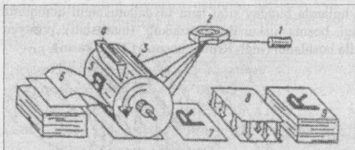
22.13-rasm. Elektronografik (lazer) printyerlarning ishlash chizmasi.
