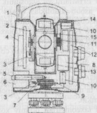
6.12-rasm. Elektron taxometr tuzilishi sxemasi
