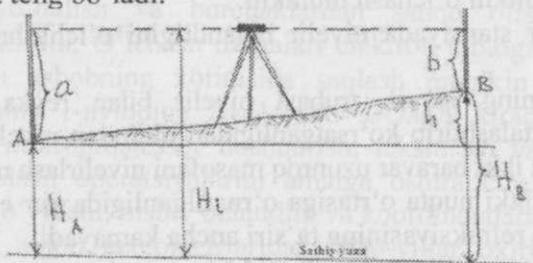
6.11-rasm. Oʻrtadan nivelirlash
