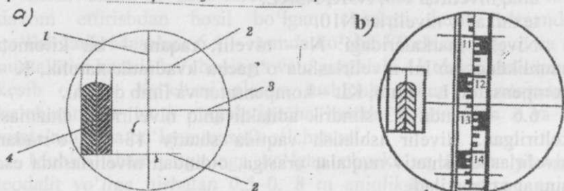
6.7-rasm. 1-vertikal ip; 2-dalnomer iplari; 3- o'rta ip; 4- silindrik adilak pufakchasinig uchlari ,bir-biriga to'g'ri keltirilgan (kontakt) holati; 6) qarash trubasida reyka tasviri
