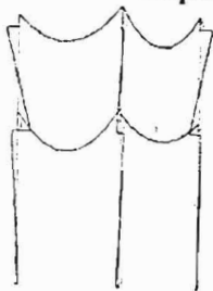
5.78- rasm. МУ eguvchi momentlar epyurasi.
