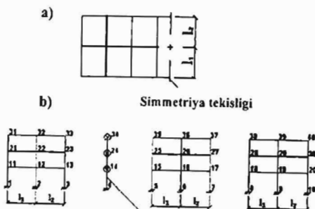
Diafragma ni modellashtiruvchi sterjen. Massalar diafragma tugunlariga to'plangan.
