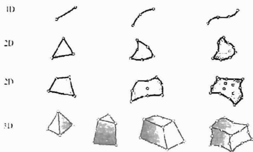
1.1-rasm. Mexanikaning bir, ikki va uch o'lchamli masalalariga mo'ljallangan chekli elementlarning asosiy turlari.
