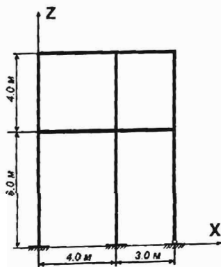
5.1-rasm. Rama sxemasi.
