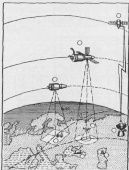
64-rasm. Tabiiy resurslarni tadqiq qiluvchi kosmik sistemalarning strukturasi.
