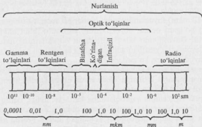
59-rasm. Aerokosmik syomkadan foydalaniladigan elektromagnit to'liqlar spektri.
