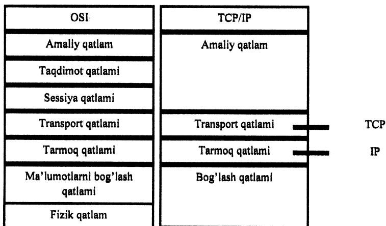
7.3-rasm. OSI va TCP/IP modellari qiyosiy ko'rinishi
