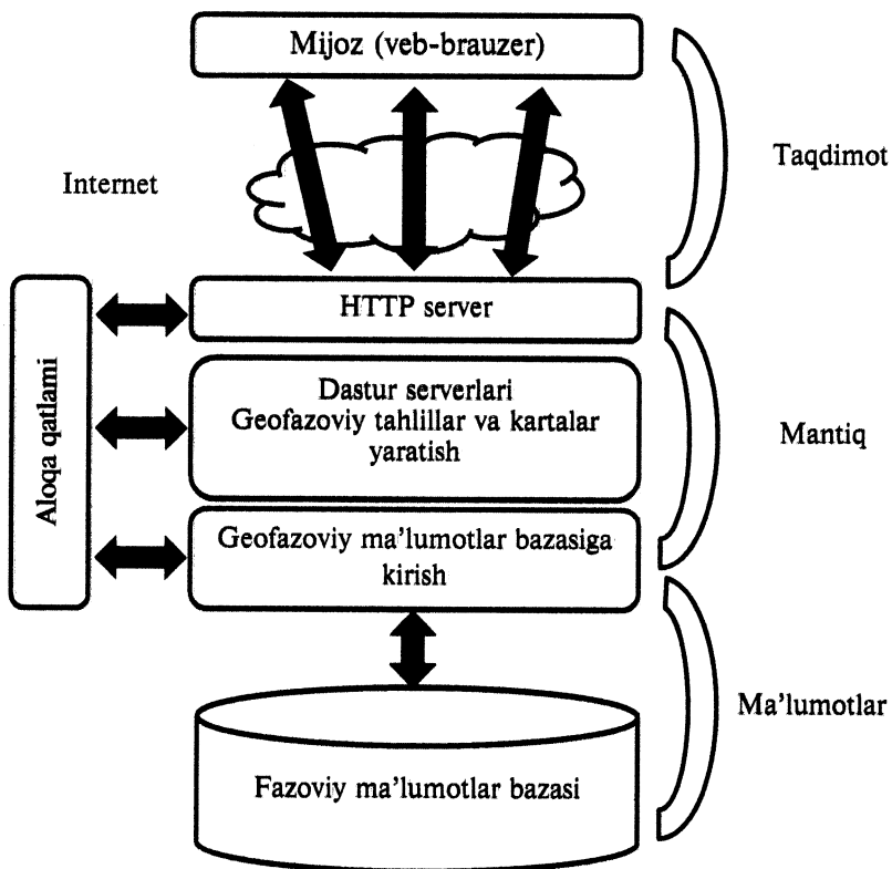
7.5-rasm. Internet GATning arxitekturalaviy mantiq diagrammasi
