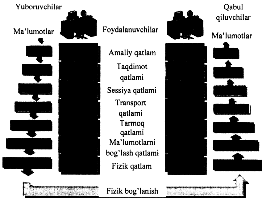
7.2-rasm. OSI modelidagi etti qatlam
