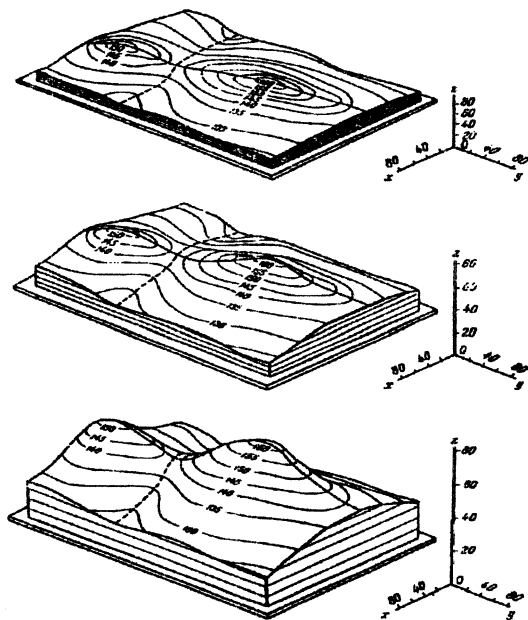
2.7-rasm. Vertikal bo‘yicha turli masshtabga ega blok-diagrammalar (Balandlik bo‘yicha tortilishi natijasida diagrammada ko‘rinmaslik joylari paydo bo‘ladi)
