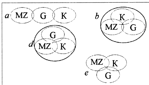
2.9-rasm. Kartografiya, geoinformatika va masofadan zondlash fanlarining bir-biri bilan bog‘liqlik modellari:
