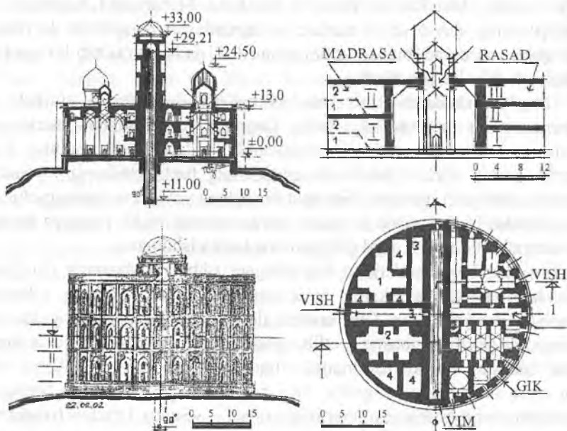
Ulug'bek rasadxonasining G.I. Korobovsev ishlagan rekonstruksiyasi.
