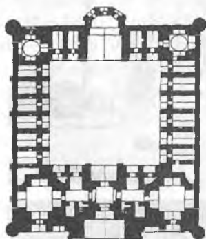
Ulug'bekning Buxoro. 1417-y. (a, b) va G'ijdivondagi. 1433-y. (d) madrasalari.
