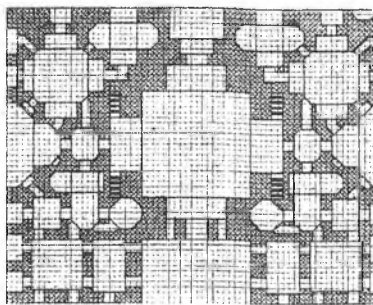
Bino tarhini ishlashda modul to'ridan foydalanish uslubi. Buxorolik me'mor chizmasi (xonaqoh). XVI asr.
