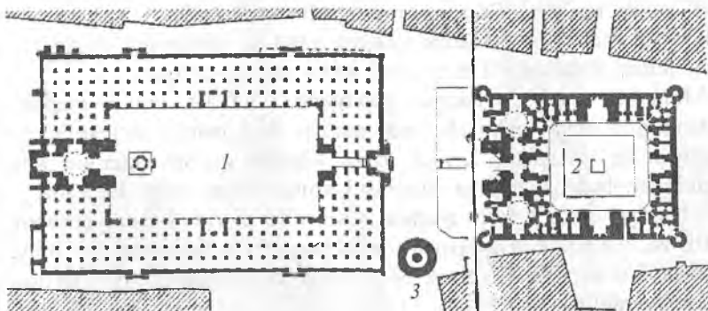
Buxoro. Poyi-Kalon ansambli tarhi.
