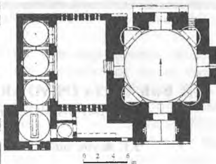
Termiz. Hakim at-Termiziy majmuasining umumiy ko'rinishi va sxematik tarhi.
