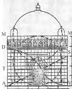
Buxoro. Somoniylar maqbarasining me'moriy chizilish uslublari (K.S. Kryukov bo'yicha). Tarhi va tarzi.
