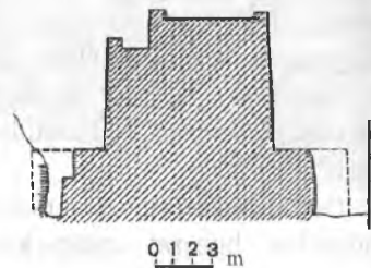
Surxondaryo viloyati. Iskandar ko'prigi tarhi va qirqimi.
