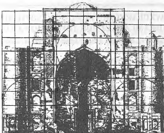
Turkistondagi Xo'ja Ahmad Yassaviy yodgorligi tarzining miqyos (modul) to'rida loyihilash tartibi.
