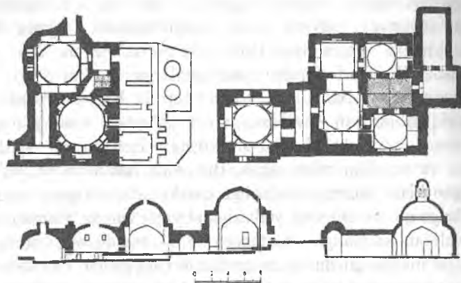
Xiva. Anushxon hammomlari tarhi va qirqimi.
