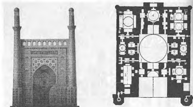
Turkiston. Xo'ja Ahmad Yassaviy majmuasi old tarzi (T.Sh Mamatmusayev rekonstruksiyasi) va tarhi (1 – qozonliq, 2 – halim xona, 3 – quduqxona, 4 – Ahmad Yassaviy maqbarasi. 5 – kitobxona, 6 – kichik Oq-saroy maqbarasi. 7 – katta Oq-saroy maqbarasi, 8 – kichik masjid. 9 – xujra).
