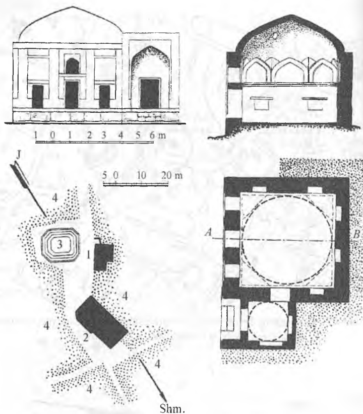
Buxorodagi Qozi Fayzi guzarining maktabi, tarxi, tarzi va qirqimi.
