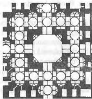
Buxoro. Toqi Zargaron savdo gumbazi. Umumiy ko'rinishi va tarhi.
