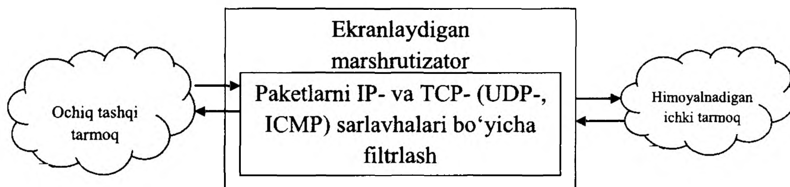
8.6-rasm. Paketli filtrning ishlash sxemasi.
