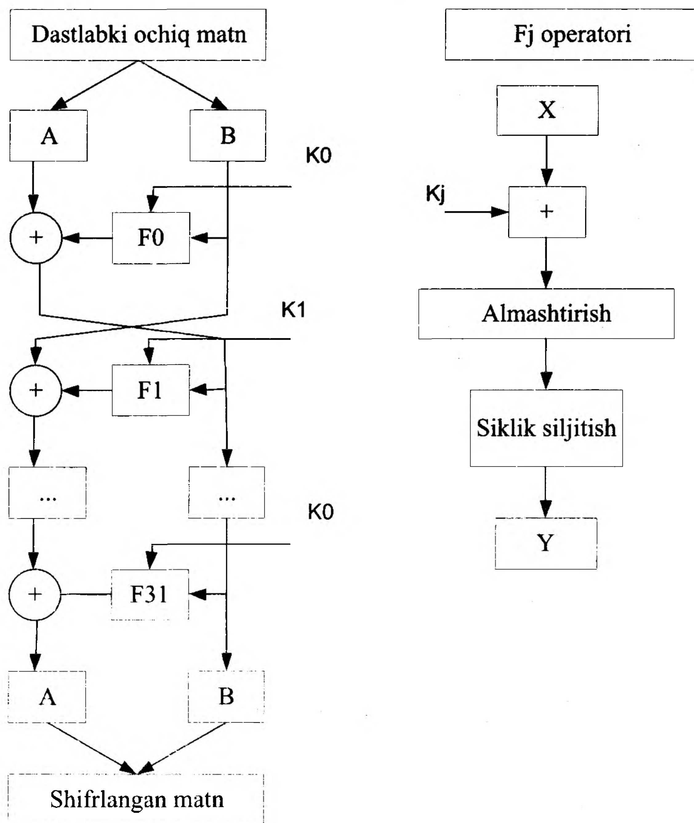
5.14-rasm. Oddiy almashtirish algoritmidagi shifrlash jarayonining blok-sxemasi.
