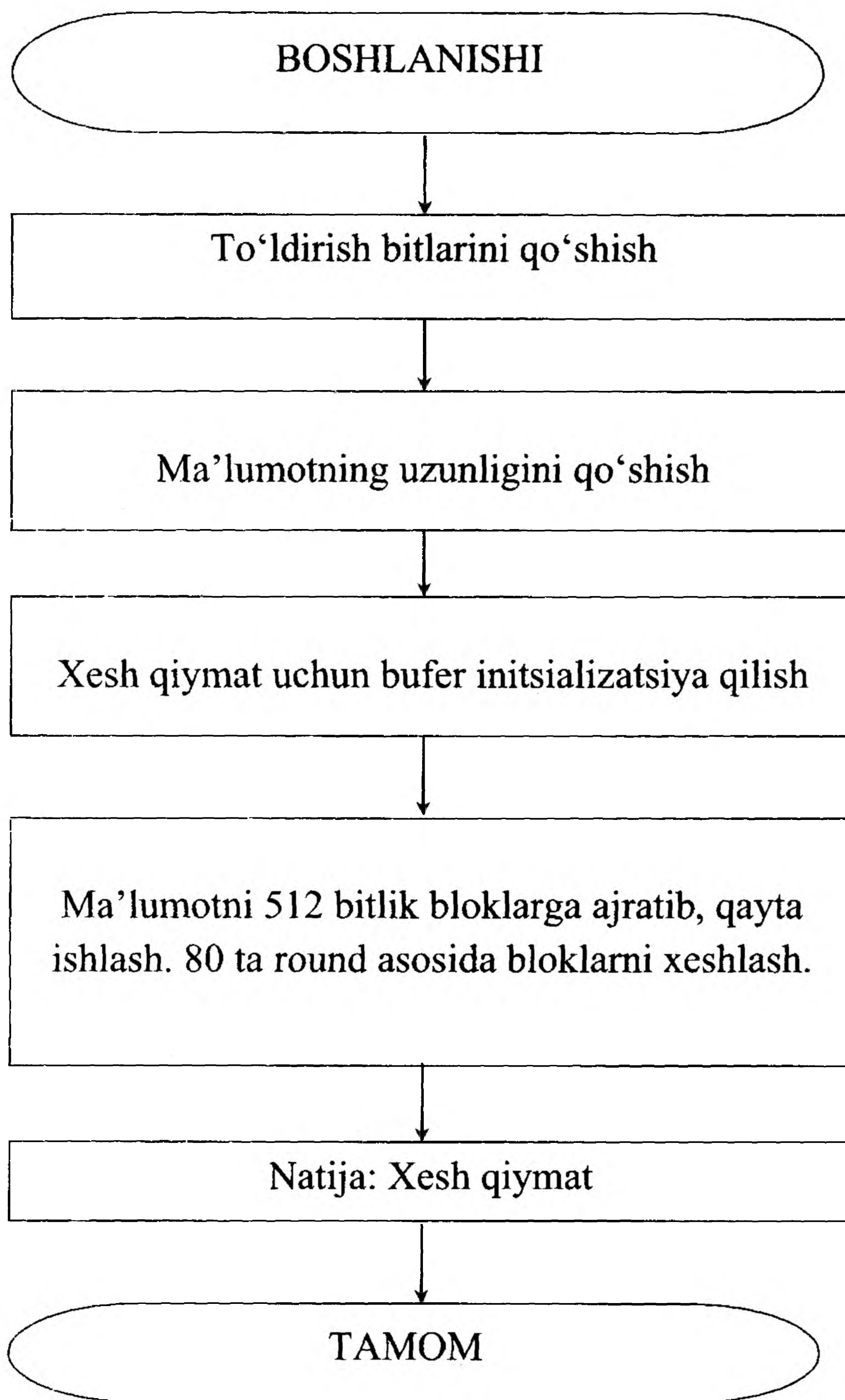
5.18-rasm. SHA1 algoritmi ishlash blok sxemasi.
