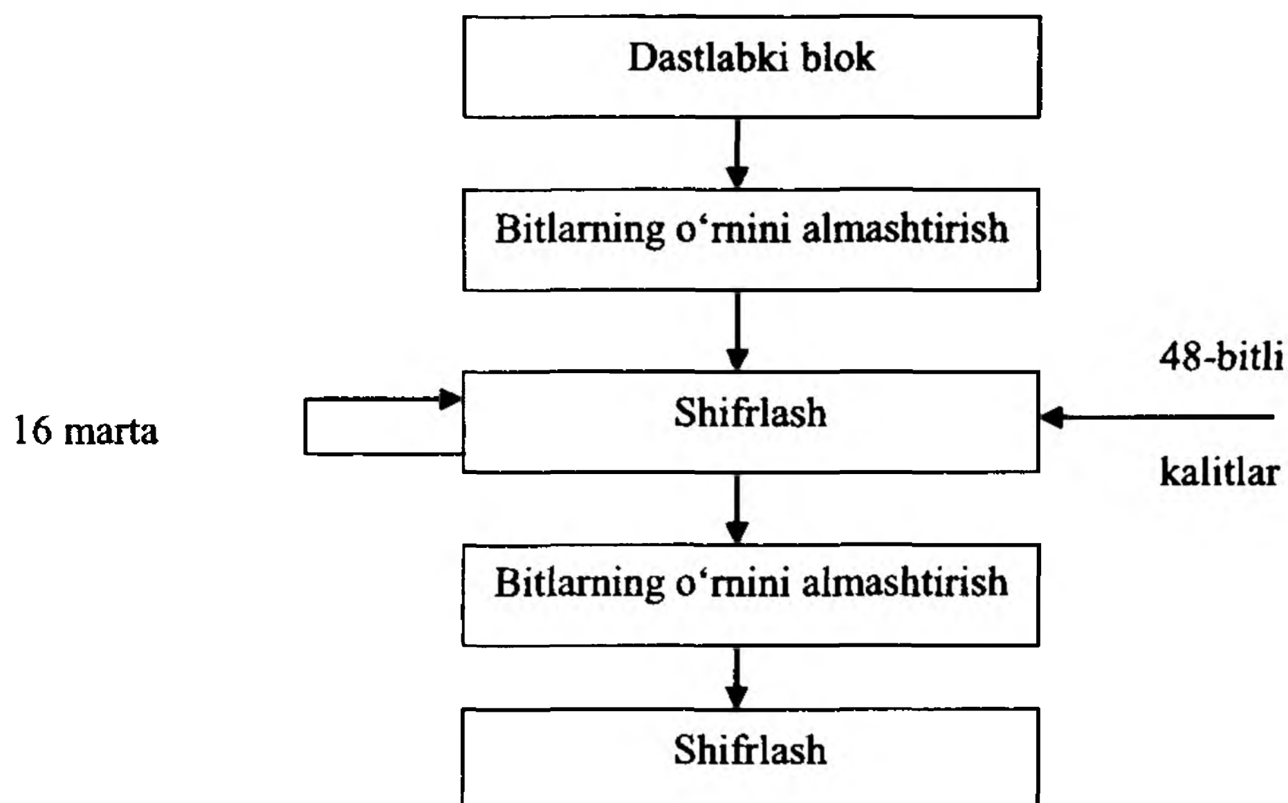
5.11- rasm. DES algoritmda shifrlash jarayonining blok-sxemasi.
