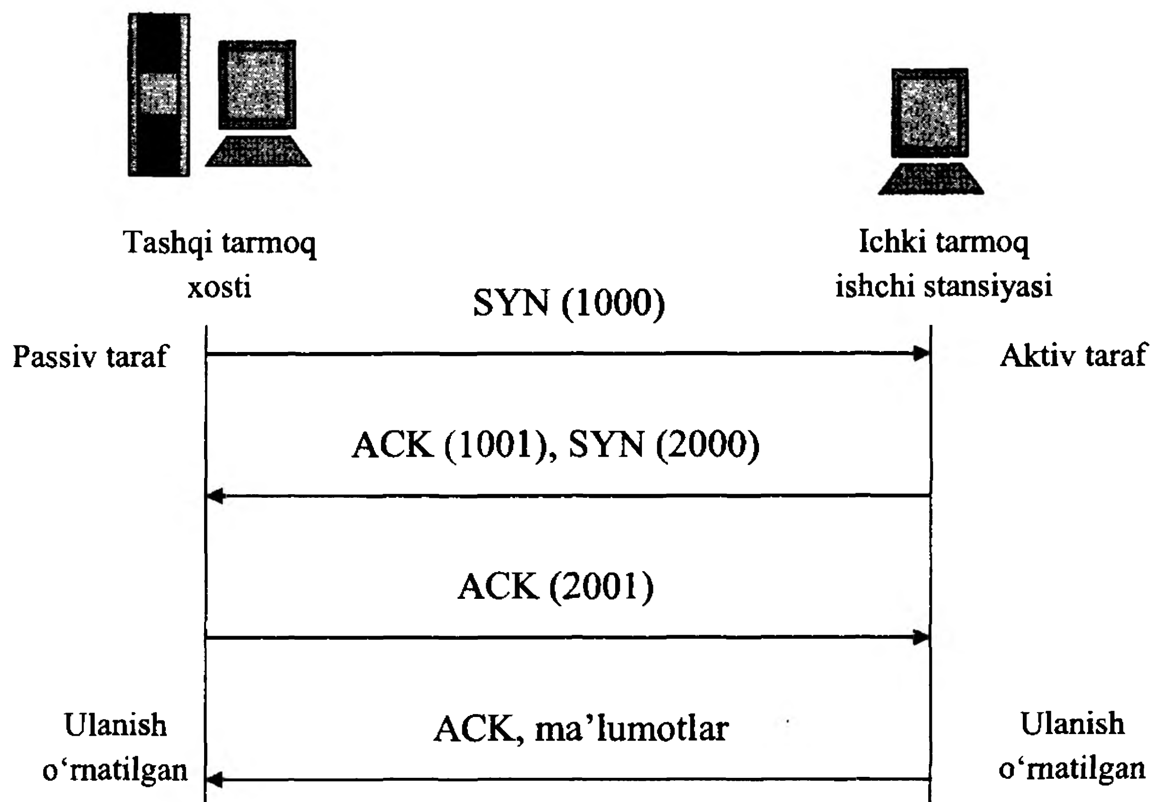
8.7-rasm. TCP protokoli bo'yicha aloqani kvitirlash sxemasi.
