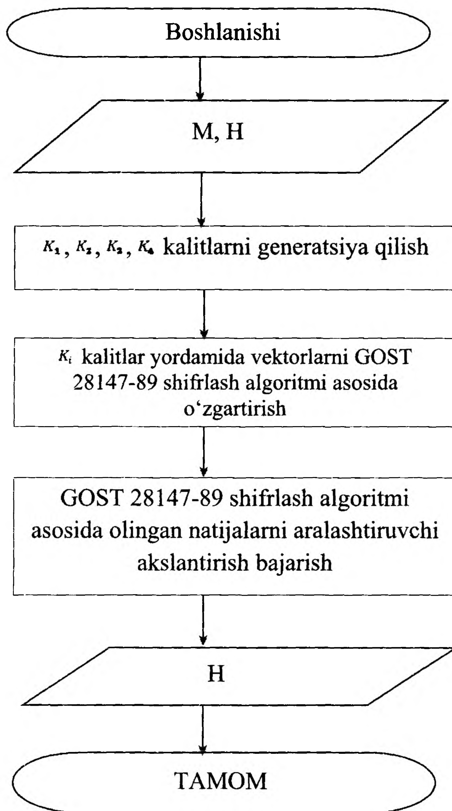
5.19-rasm. Xesh qiymatni hisoblash algoritmining blok-sxemasi.
