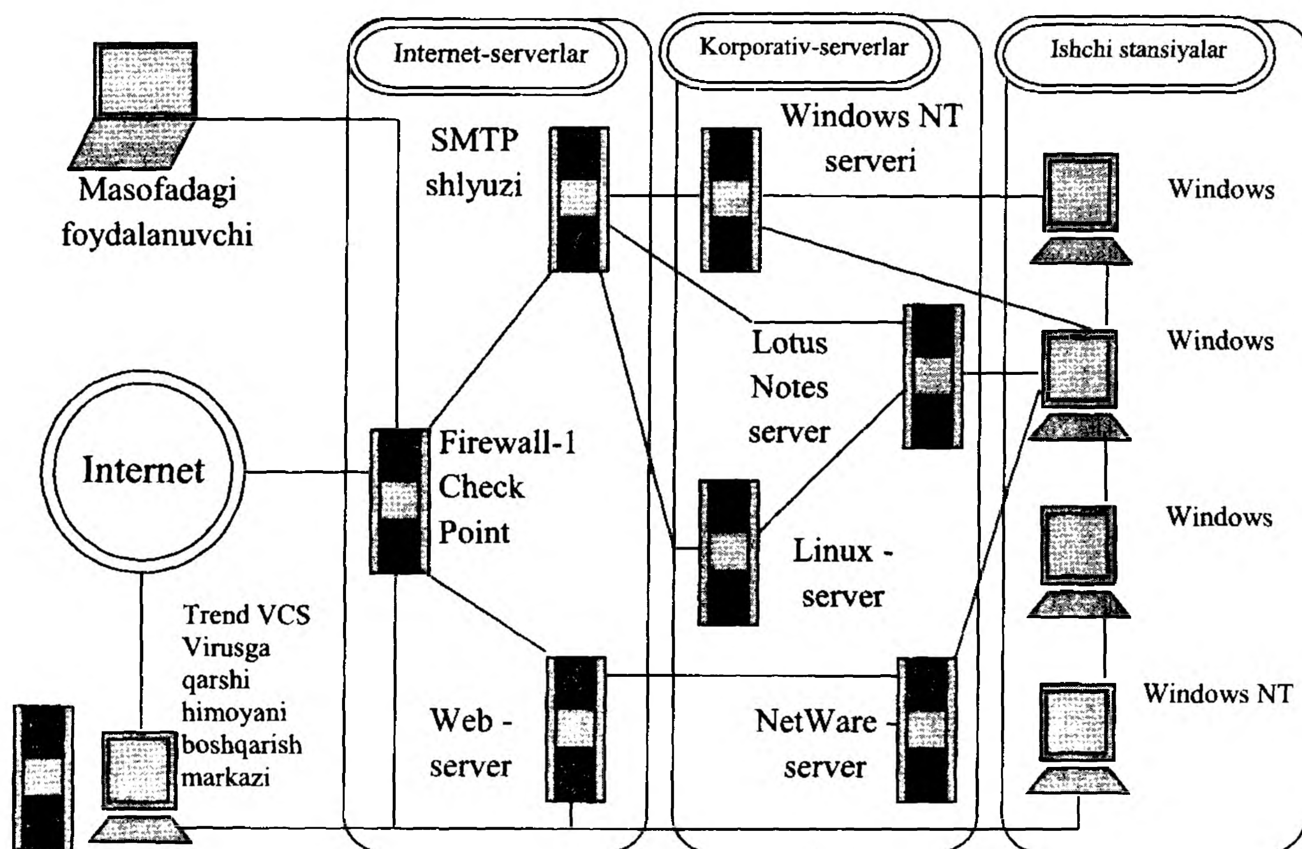
7.2-rasm. Korporativ tarmoqning namunaviy arxitekturasini.
