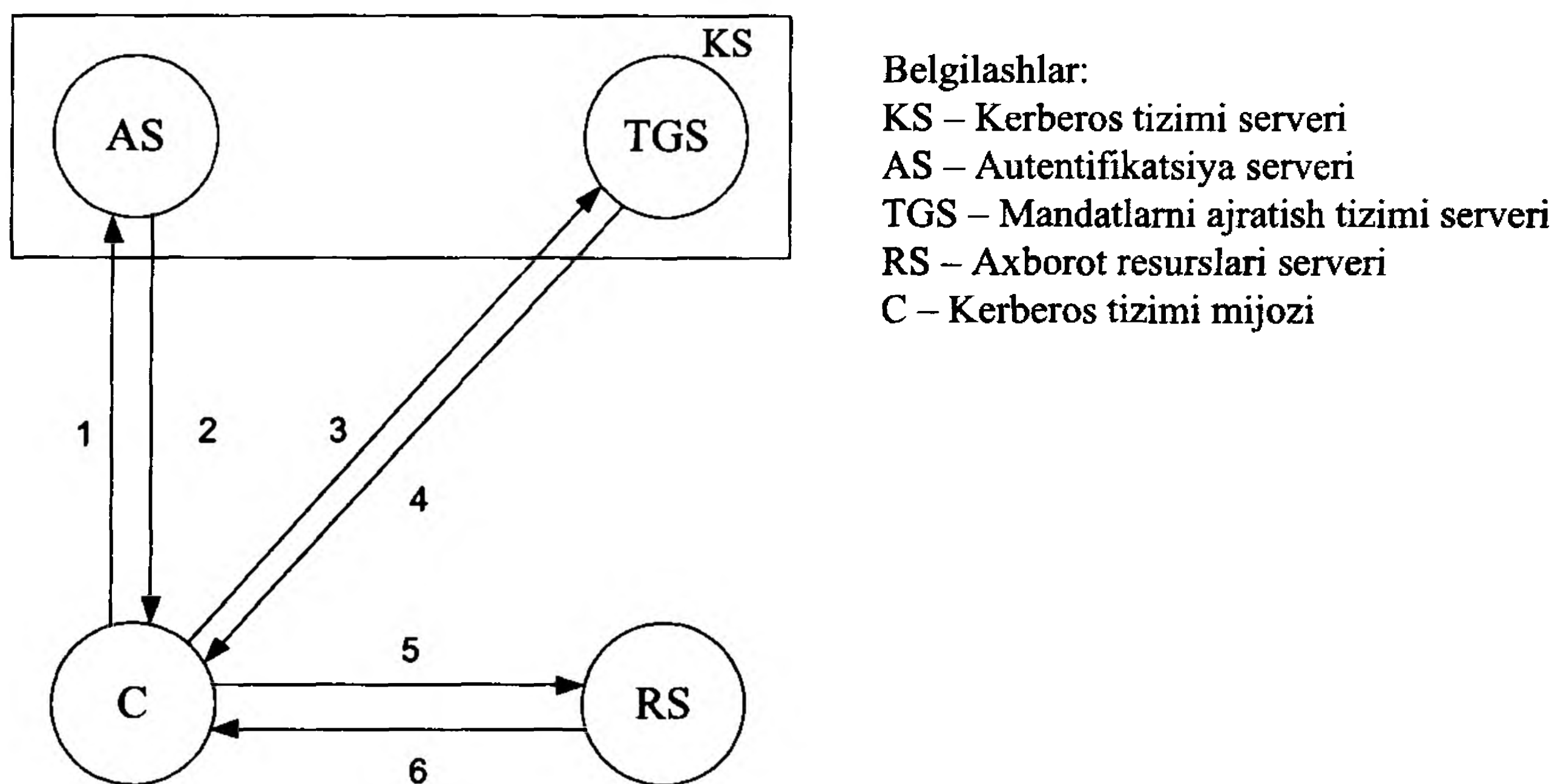
6.2-rasm. Kerberos protokolining ishlash sxemasi.
