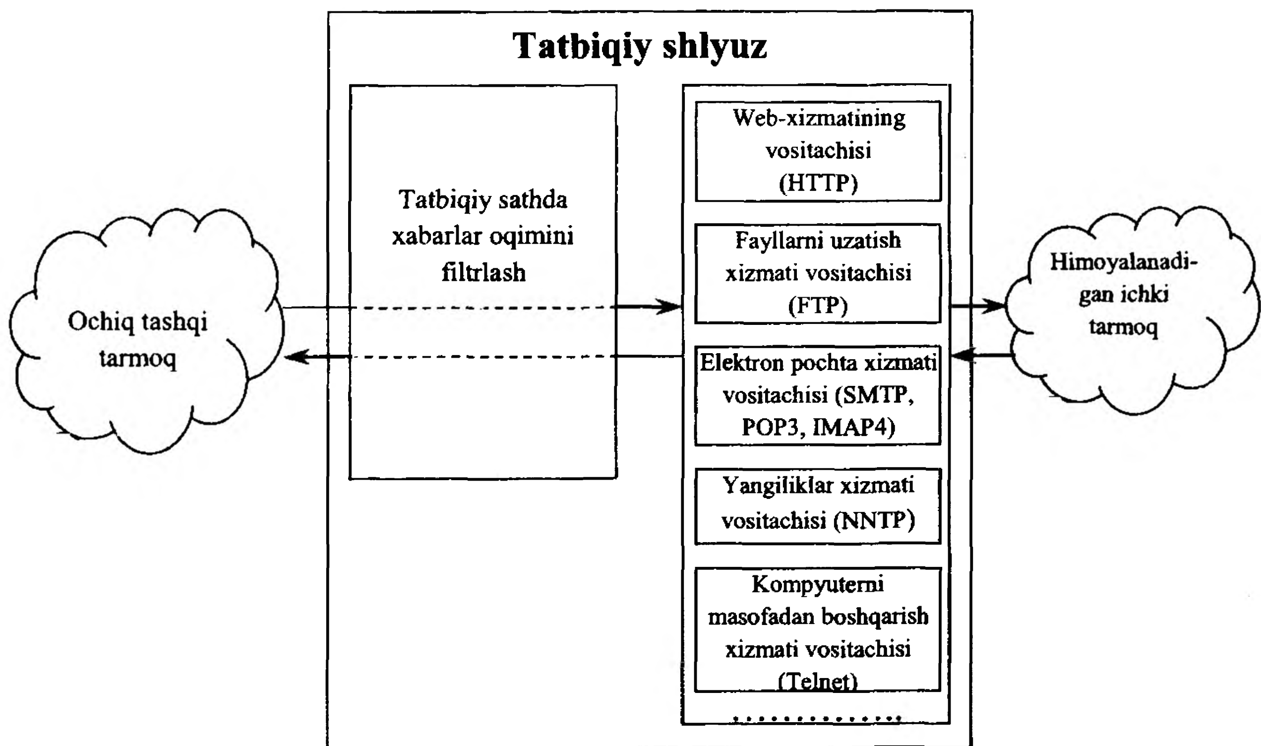
8.9-rasm. Tatbiqiy shlyuzning ishlash sxemasi.
