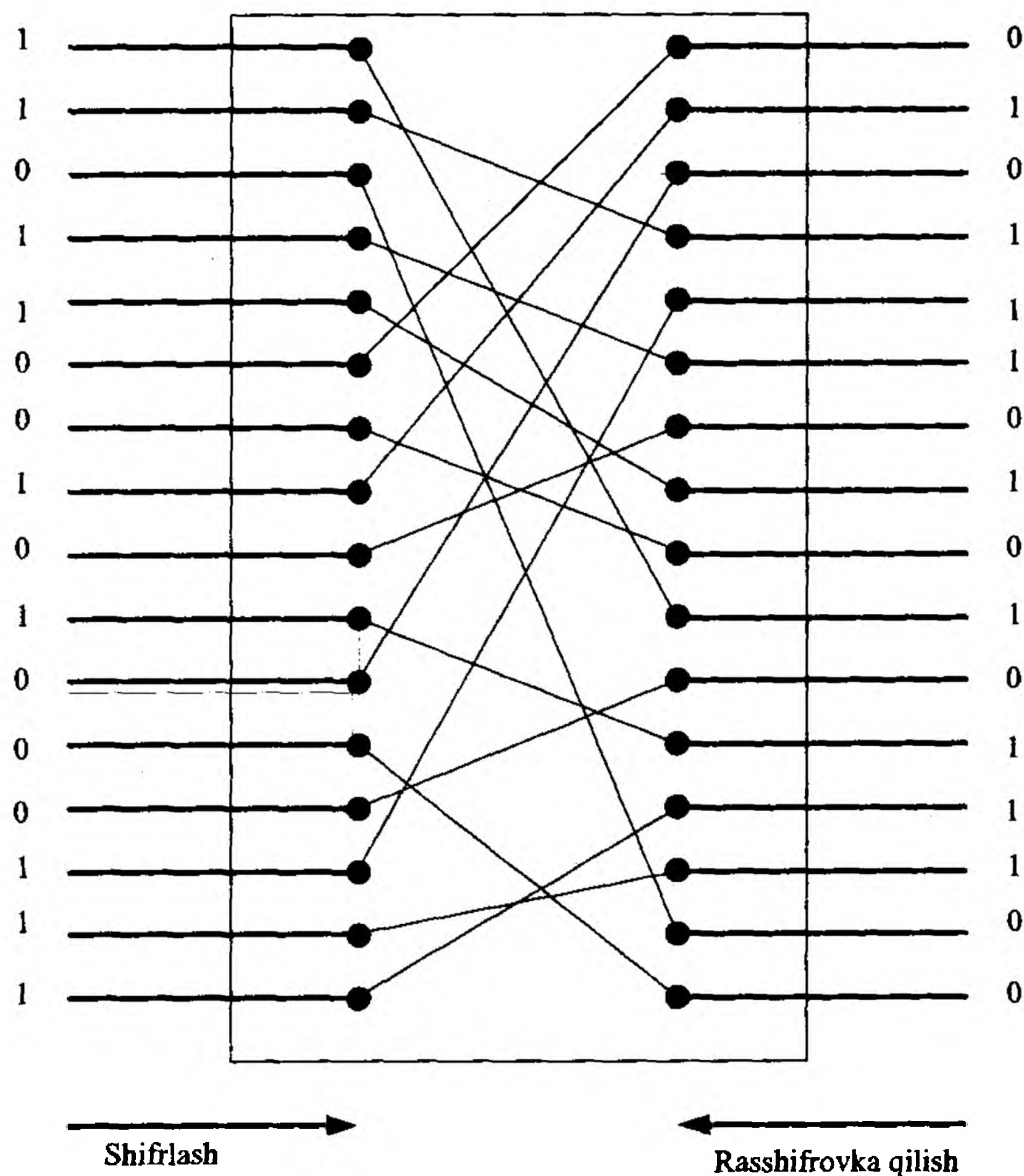
5.7-rasm. O‘rin almashtirish sxemasi.
