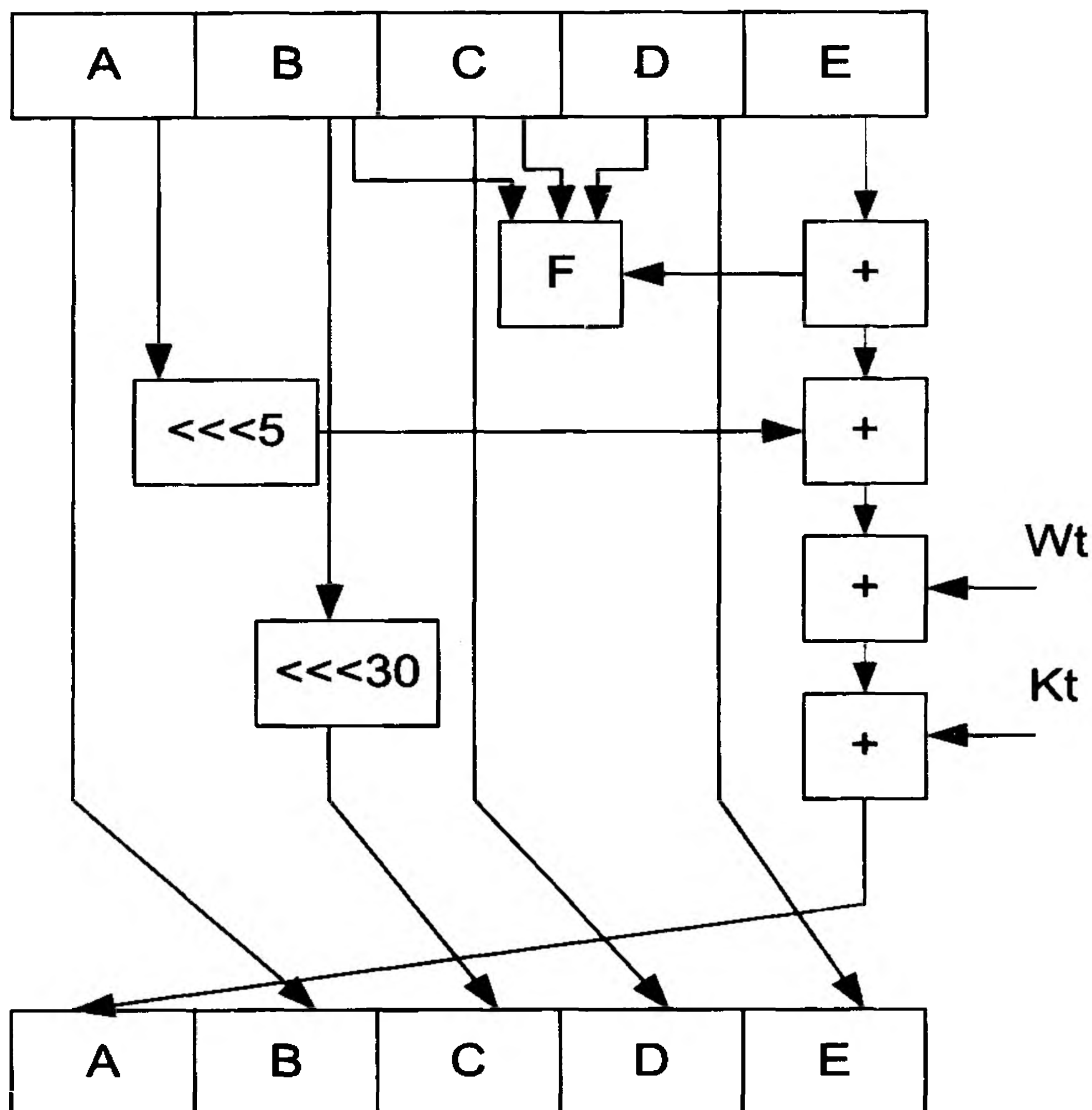
5.17-rasm. SHA-1 algoritmidagi bir iteratsiyasining sxemasi.
