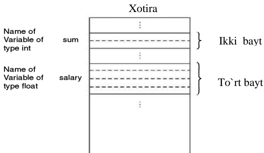
12.8-rasm. Xotiradagi int va float turidagi o`zgaruvchilar
