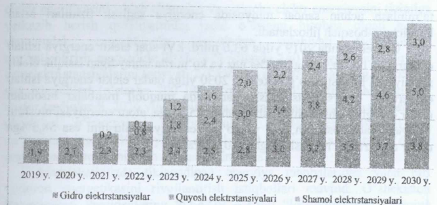
10.3.1-rasm. O'zbekistonda 2030 yilga qadar muqobil energiya asosida elektr energiya ishlab chiqarish quvvatlarini o'rnatishning prognoz ko'rsatkichlari, MVt 309
