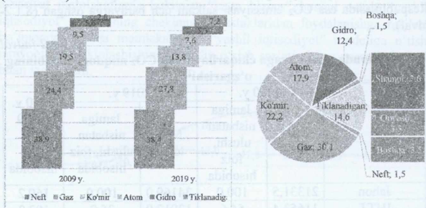
8.1.2-rasm. IHTT mamlakatlarida birlamchi energiya iste'moli tarkibining o'zgarishi, %.
