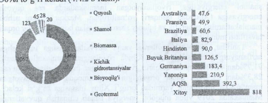
4.5.2-rasm. 2010-2019 yillarda tiklanadigan energiya quvvatlarini ishga tushirish uchun sarflangan jami investitsiyalar miqdori, mlrd. doll 116 .
