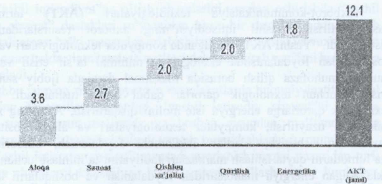
2.4.1-rasm. Axborot-kommunikatsiya texnologiyalarining 2030 yilga qadar issiqxona gazlarini chiqarish hajmini qisqartirishga qo'shadigan potensial hissasi, mlrd. tonna CO 2 ekvivalentida 46
