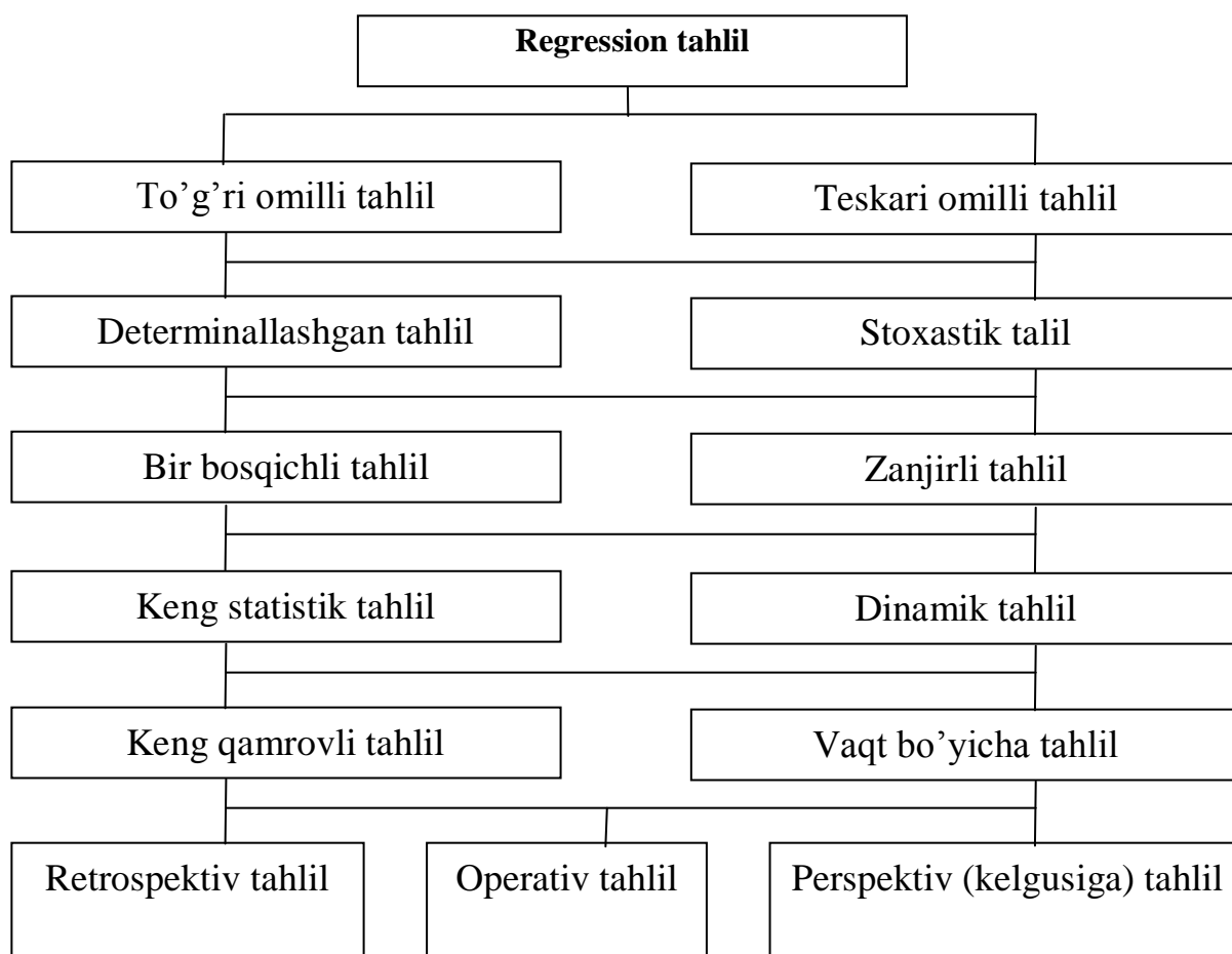
3.1-rasm. Regression tahlilning masalalar tavsifining umumlashgan sxemasi
